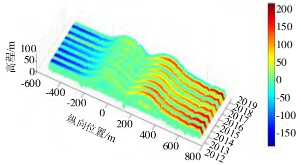
图 7 2012 年~2019 年大桥变形(mm)
