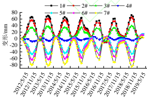
图 6 支座变形时间序列
