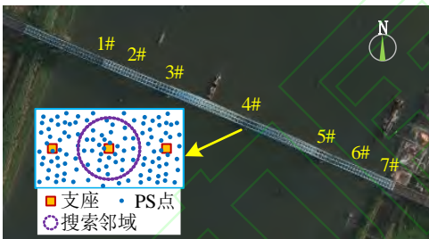
图 5 支座布置
