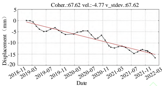
(c) 时间段 II 内目标点 B 变形时间序列
