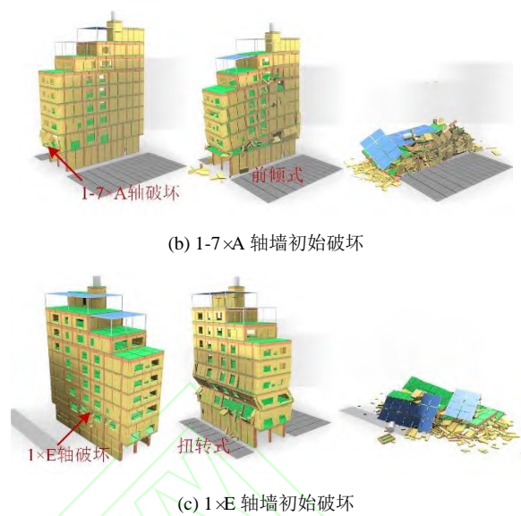
图 18 不同部位构件失效后倒塌效果
