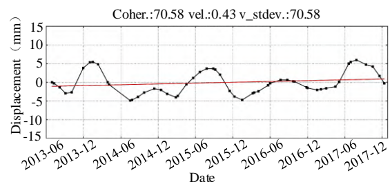
(a) 时间段 I 内目标点 A 变形时间序列
