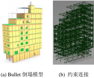
图 14 Bullet 倒塌模型与约束连接
