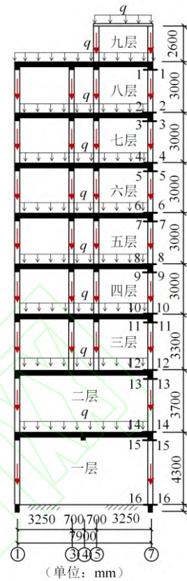
图 9 荷载传递路径示意图
