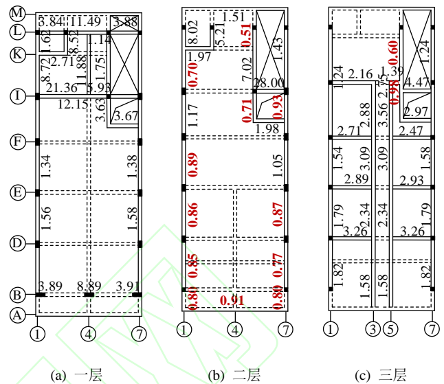
图 7 底部三层砌体墙抗力与效应值比
