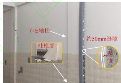
图3 倒塌前二层东侧墙柱破损征兆示意图
