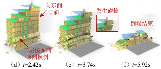
图 15 仿真模拟结构倒塌全过程
