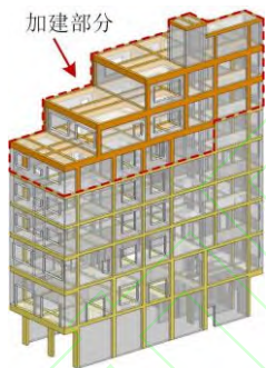
图 6 结构静力计算分析模型
