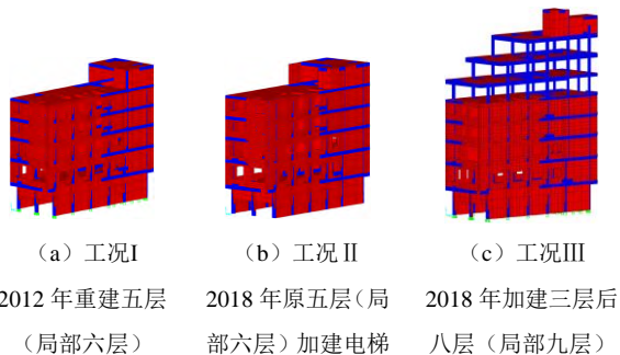
图10 各工况下SAP2000计算模型
