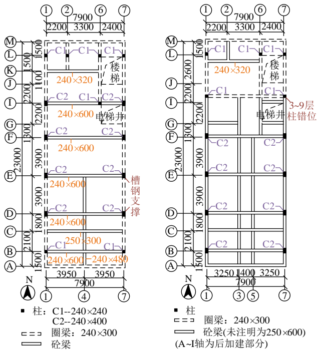
(a) 结构二层 (b) 结构六层
