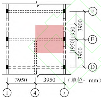
图 8 计算单元
